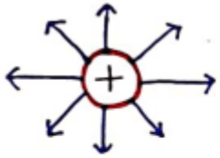
(i) धनावेश की वैद्युत बल रेखाएँ
